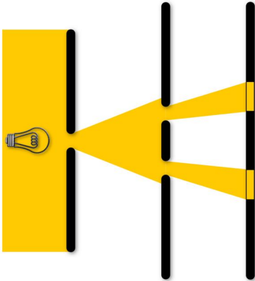
Strahlenmodell
