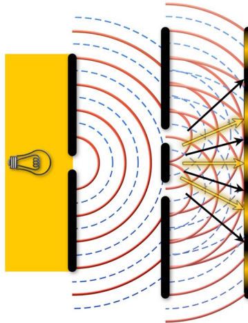
Wellenmodell
